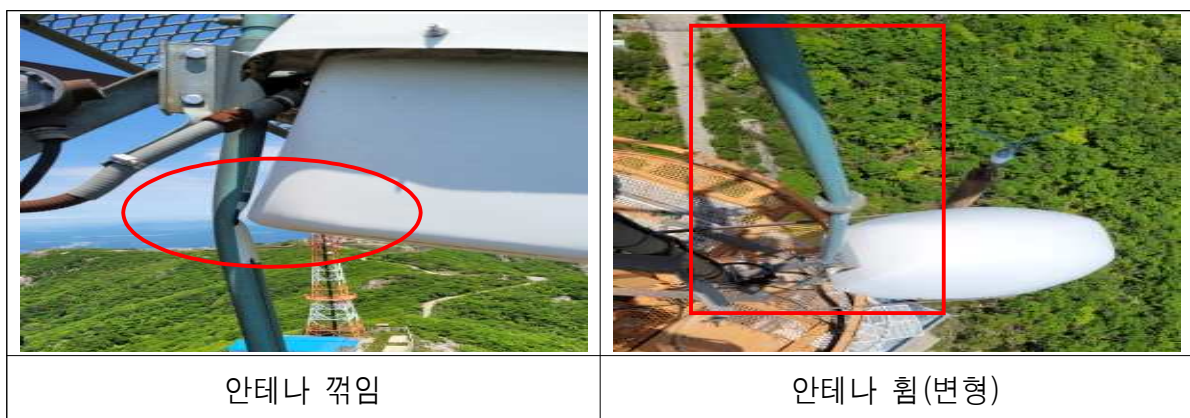
[사진 1] 팔공산 송신소 안테나 손상 모습
